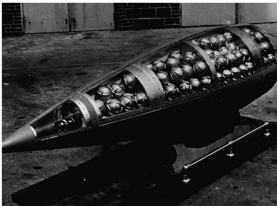
Kovinė raketos galvutė su nervus paralyžiuojančių cheminių medžiagų užtaisais
