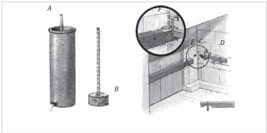
Liūto Vartų Milete skląstis ir spyna. Skląstis (A) išstumiamas iš lizdo priešingoje sienoje (B) ir įstumiamas į ertmę (C). Velkė (D) užstumiama ant skląščio A ir įtvirtinama ertmėje (E). Po to į jungties vietą įkišamas spynos kaištis (F), kuris tvirtai sujungia sklendę ir skląstį
