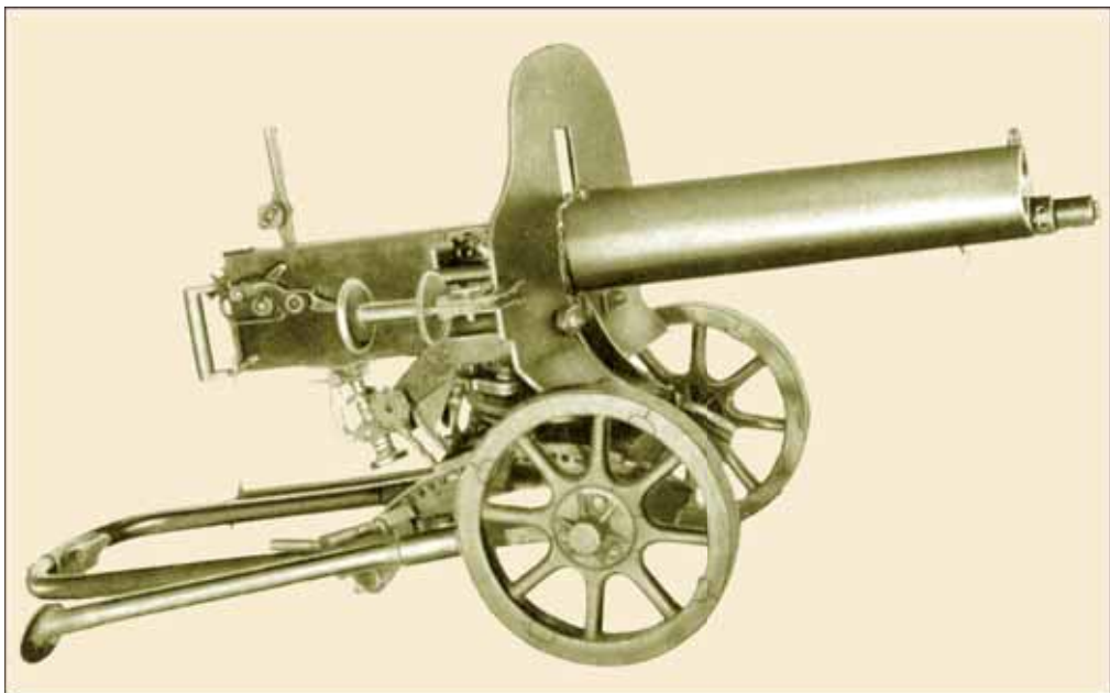
13. Sunkusis kulkosvaidis „Maxsim 1910“ (1910 m. modelis, kalibras – 7,62 mm, bendras ilgis – 1067 mm, bendras svoris – 66 kg, juostos talpa – 250 šovinių, greitašauda – 250–300 šovinių per minutę, šalis gamintoja – Rusija). VDKM. G-34
