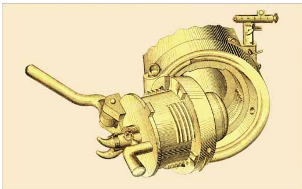
30. Lengvojo artilerijos pabūklo stūmoklinės spynos brėžinys. Чертежи к краткому руководству артиллерической службы с полевыми пушками. С. Петербург. 1897
