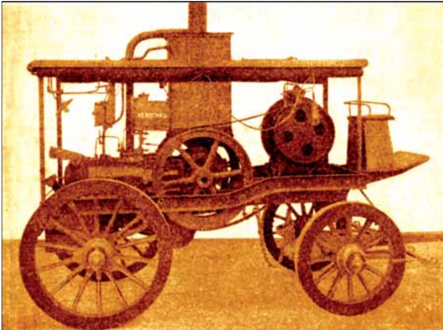
56. Benzininė lauko elektros stotis. XIX a. pab.–XX a. pr. Энциклопедический словарь. Т. XL a . С. Петербург. 1904
