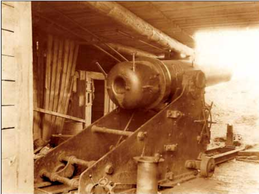
35. Kauno tvirtovės 152 mm, 190 pūdų patranka dengtoje stacionariojoje pozicijoje. 1915 m. P. Butkevičiaus archyvas
