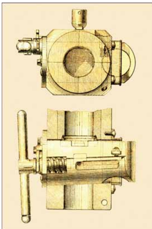
29. Lengvojo artilerijos pabūklo pleištinės spynos brėžinys. Чертежи к краткому руководству артиллерической службы с полевыми пушками. С. Петербург. 1897
