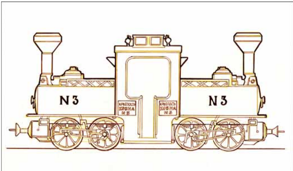
62. Kauno tvirtovės siaurojo geležinkelio aštuonių ašių tanko-garvežio „Pežo Bordon“ brėžinio rekonstrukcija. XIX a. pab. KAA
