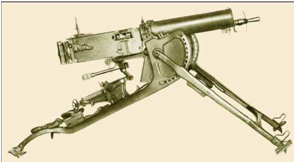
24. Sunkusis kulkosvaidis MG-08 (1908 m. modelis, kalibras – 7,92 mm, bendras ilgis – 1187 mm, masė – 58 kg, juostos talpa – 250 šovinių, greitašauda – 250–300 šovinių per minutę, šalis gamintoja – Vokietija). VDKM. G-33
