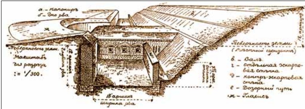
1. Forto centrinio kaponieriaus piešinys. Энциклопедический словарь. Т. XIV. С. Петербург. 1895
