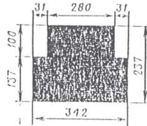
17 pieš. TANKAS (16 taikinys)
