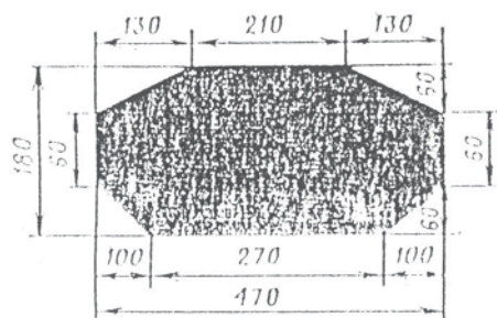
21 pieš. ŠARVUOTIS (20 taikinys)
